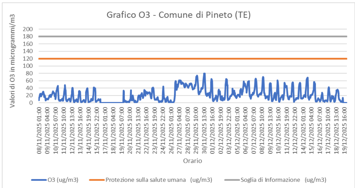
Fig. 9 profilo temporale dei livelli di Ozono (valori medi orari) rilevati durante la campagna di Pineto (TE). La linea arancione indica il valore medio annuale da non superare. La linea grigia il valore della “Soglia di informazione al pubblico”.
